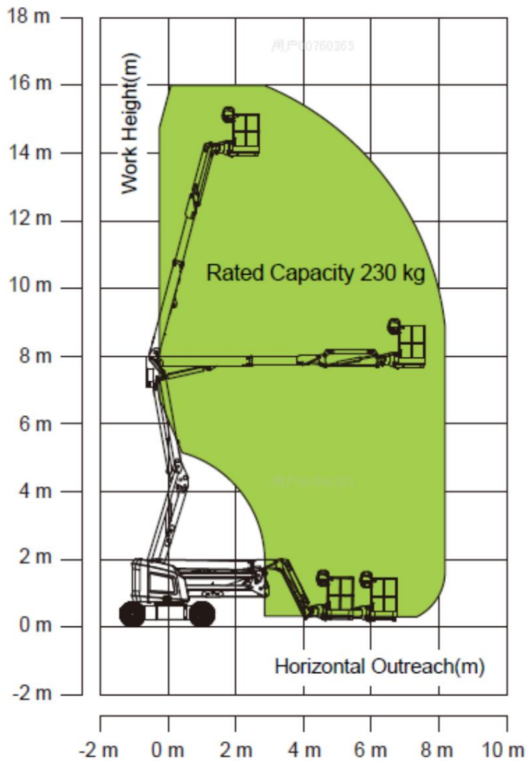
Figura 7-1 Gama de mișcare ZA14NJE-Li
