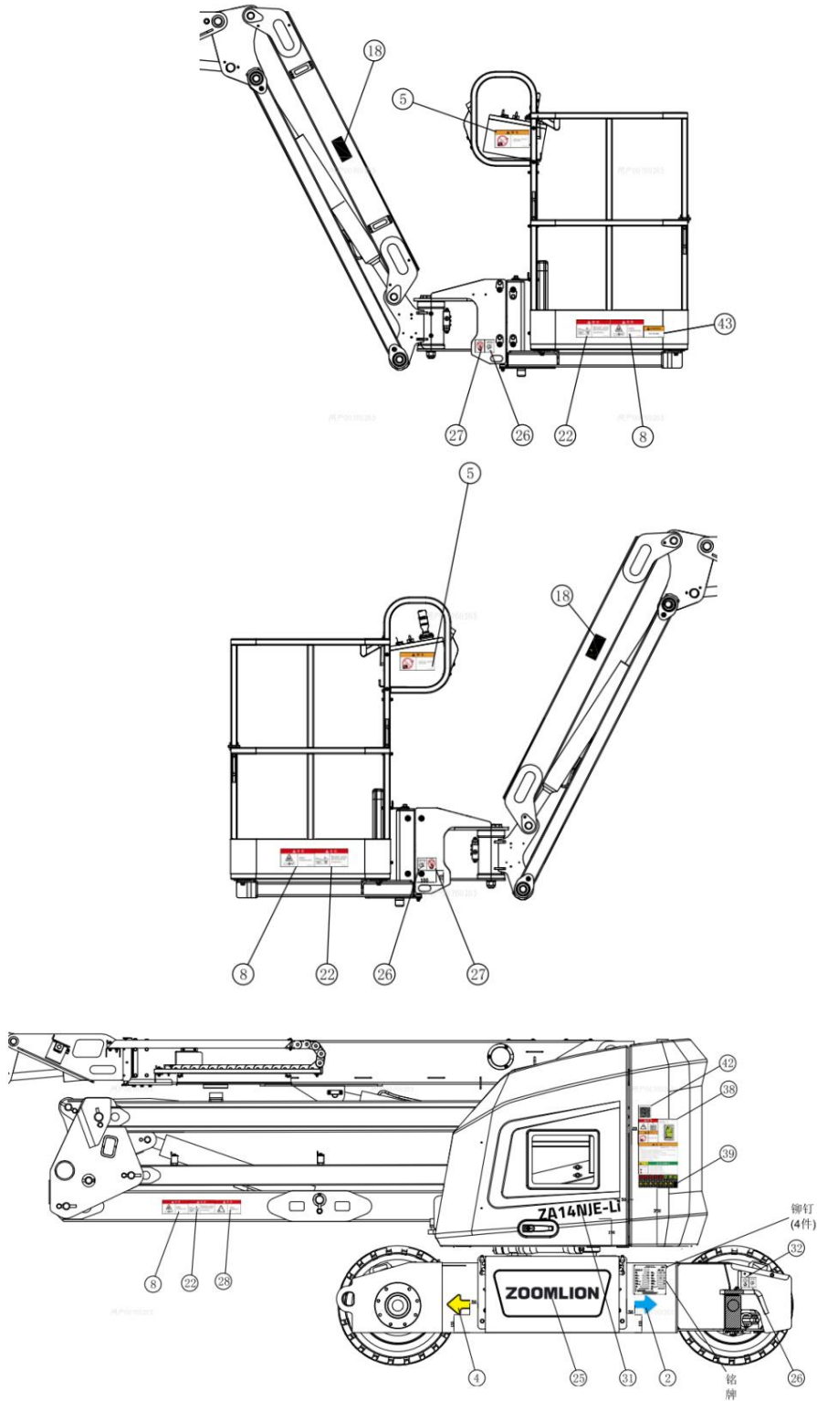
Figura 3-1 Poziția decal (continuu)
