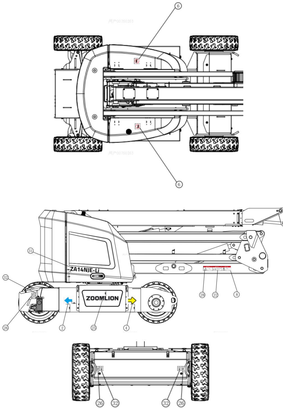
Figura 3-1 Poziția decal (continuu)
