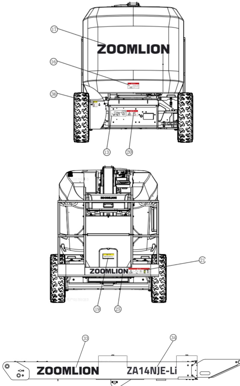
Figura 3-1 Poziția decal (continuu)
