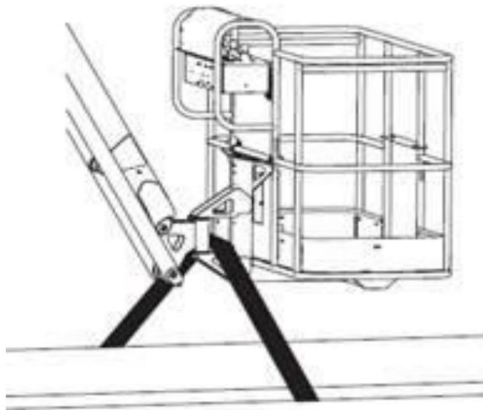
Figura 4-6 Securizarea platformei
