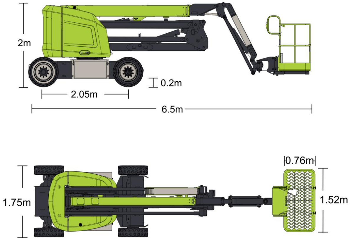
Figura 7-2 Dimensiunea ZA14NJE-Li în modul de călătorie
